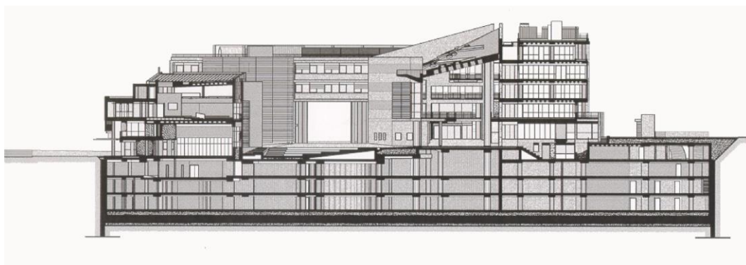
ΧΑΡΑΚΤΗΡΙΣΤΙΚΕΣ ΤΟΜΕΣ ΣΥΓΚΡΟΤΗΜΑΤΟΣ
