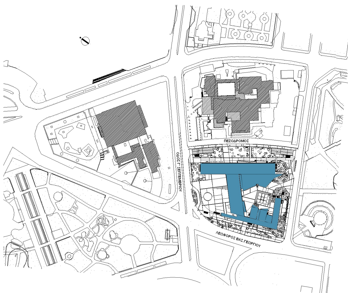
ΤΟΠΟΓΡΑΦΙΚΟ ΔΙΑΓΡΑΜΜΑ
